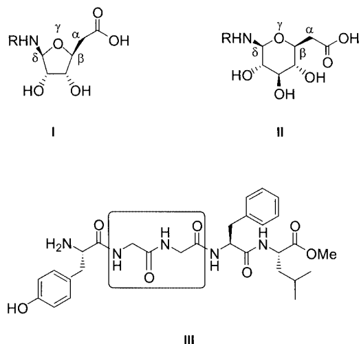
Figure 1. Furanoid \delta -SAA I , pyranoid \delta -SAA II and Leu-enkephalin III
